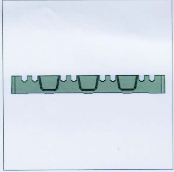
1.2 4X2F Bara Mesnet İzolatörü
